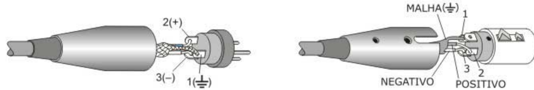
Figura A: Conectores XLR
